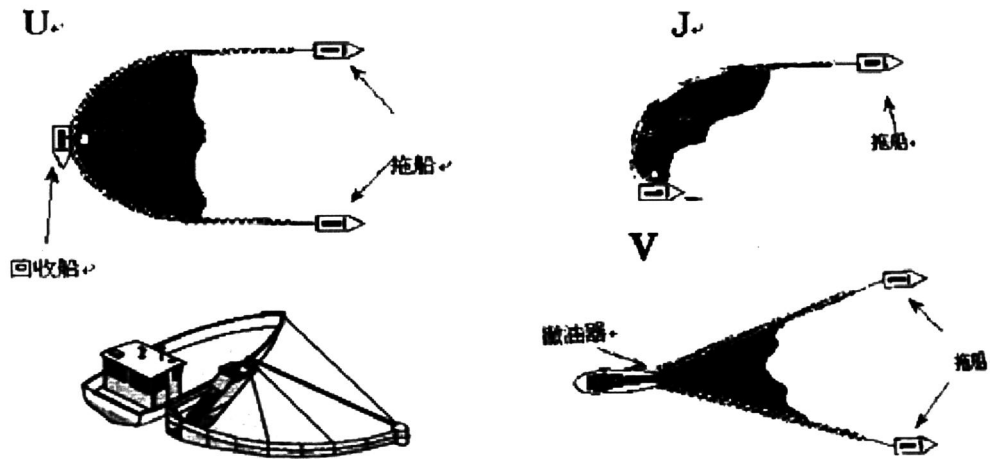
图 5-1 清除作业方式
