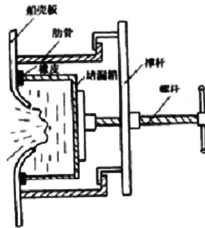
图 3-3 堵漏箱及使用方法
